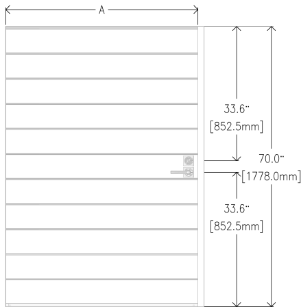
ELEVACIÓN — FRENTE
